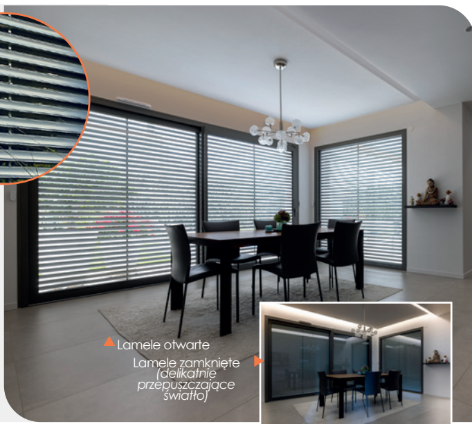
Pozycja wentylacyjna Pozycja doświetlająca Pozycja zaciemniająca
